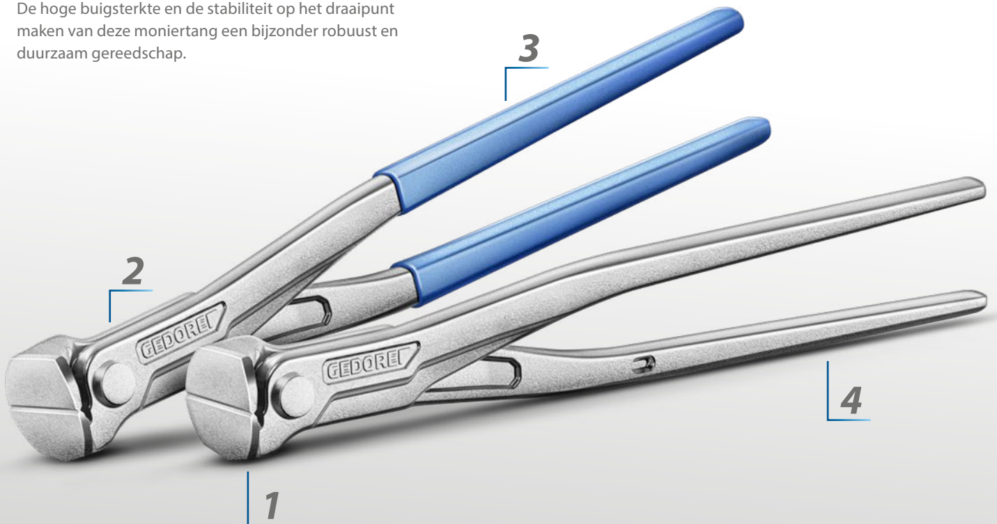
Moniertangen - 8380 L
