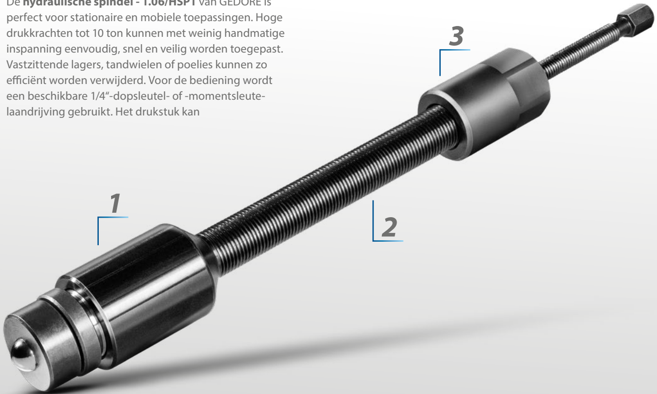
Hydraulische spindel -1.06/HSP1
